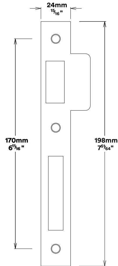
Striker Plate
